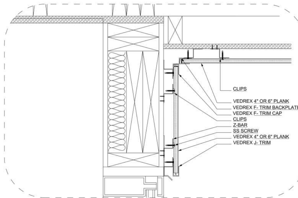
D DETAIL S-08 SCALE: 1.0" 2.0" 5.0"
