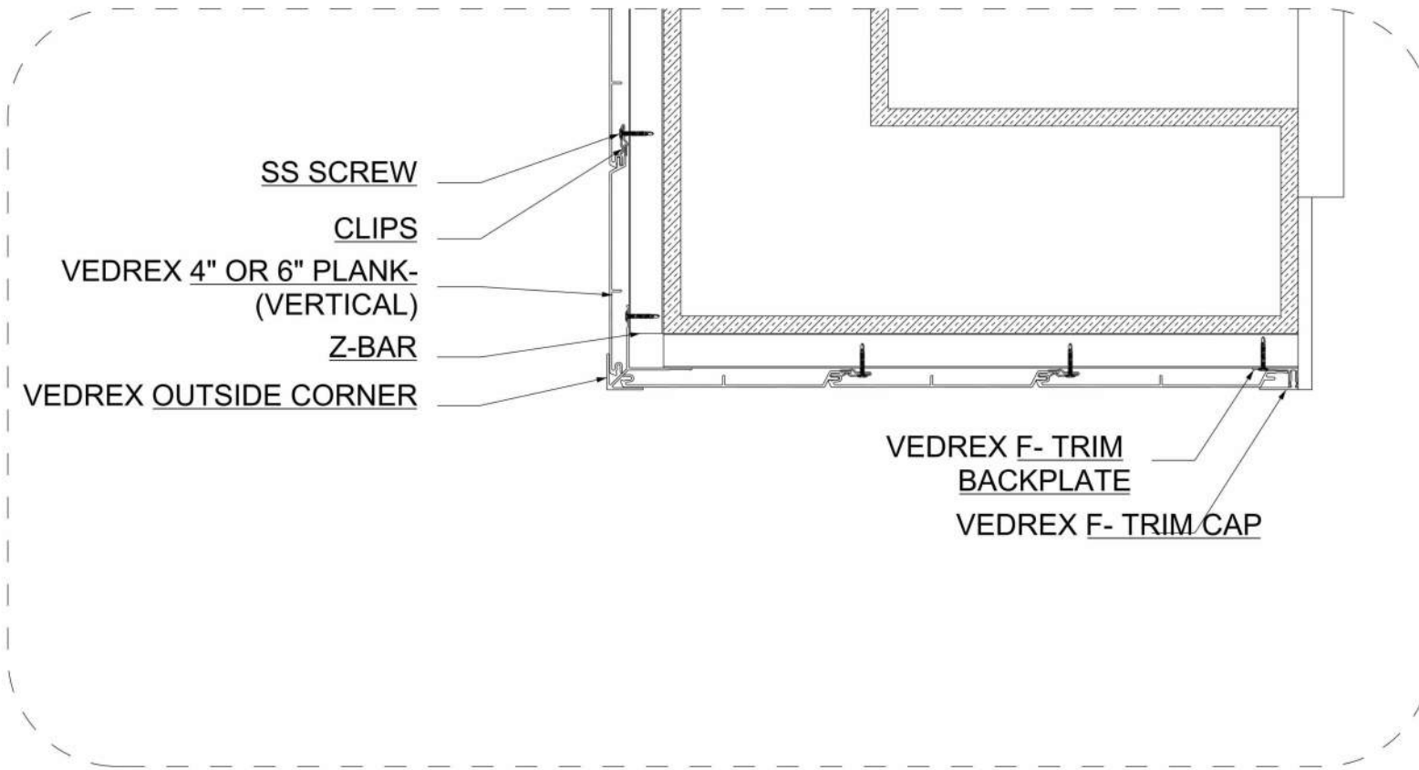
D ETAIL D-03
