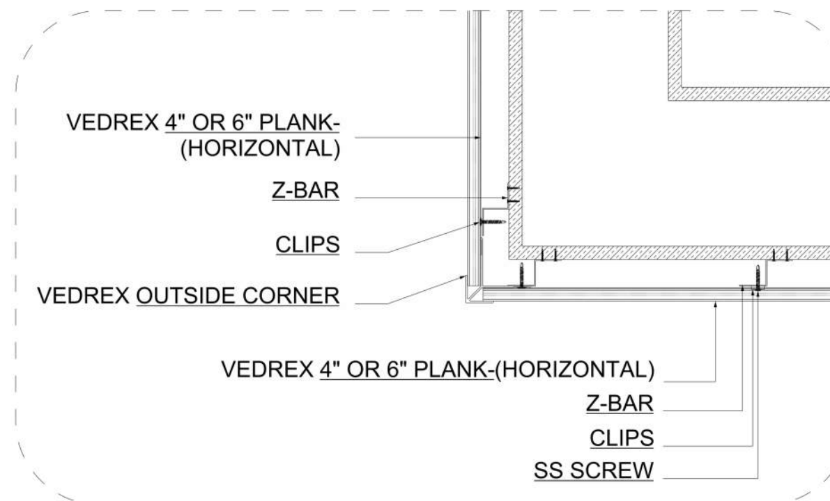
D DETAIL D-09 SCALE:
