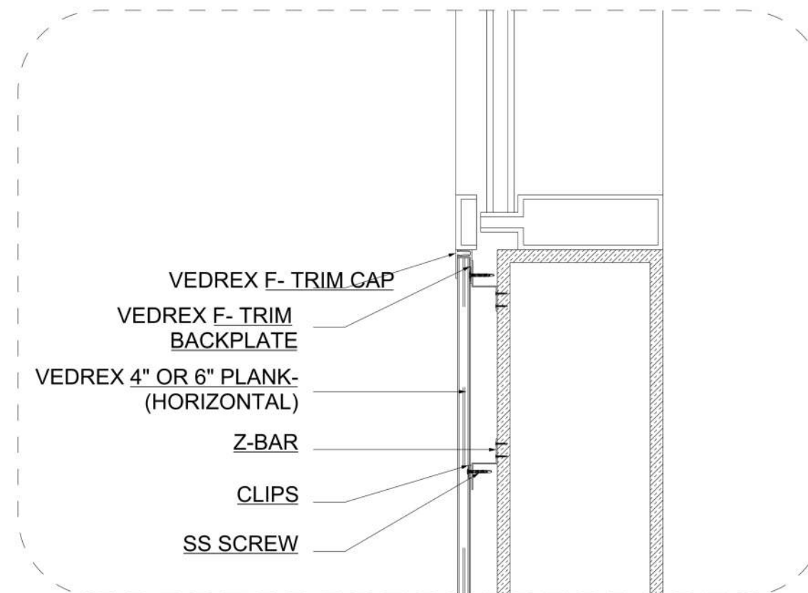
D DETAIL D-08 SCALE:
