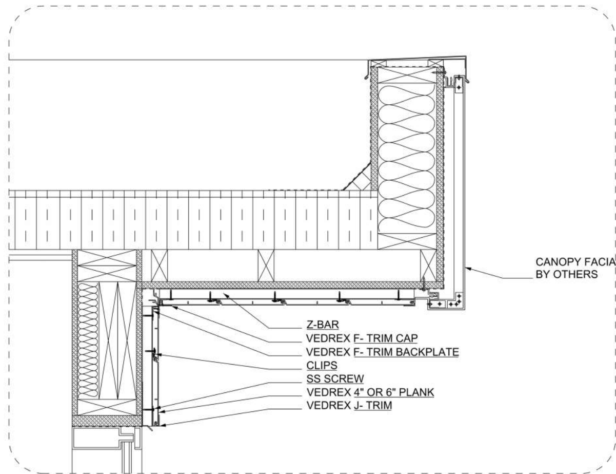
D DETAIL S-07 SCALE: 1.0" 2.0" 5.0"
